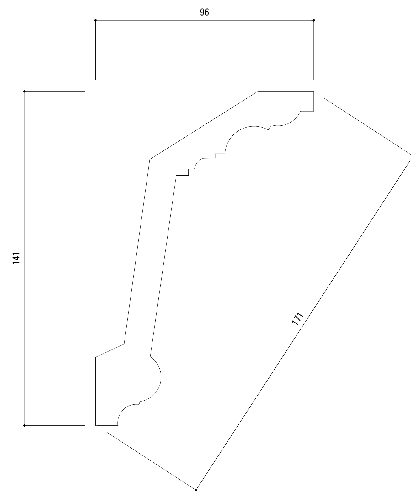
NMG005 141×96×171 ※ ポリウレタン製のため、若干の寸法誤差がある場合があります。
