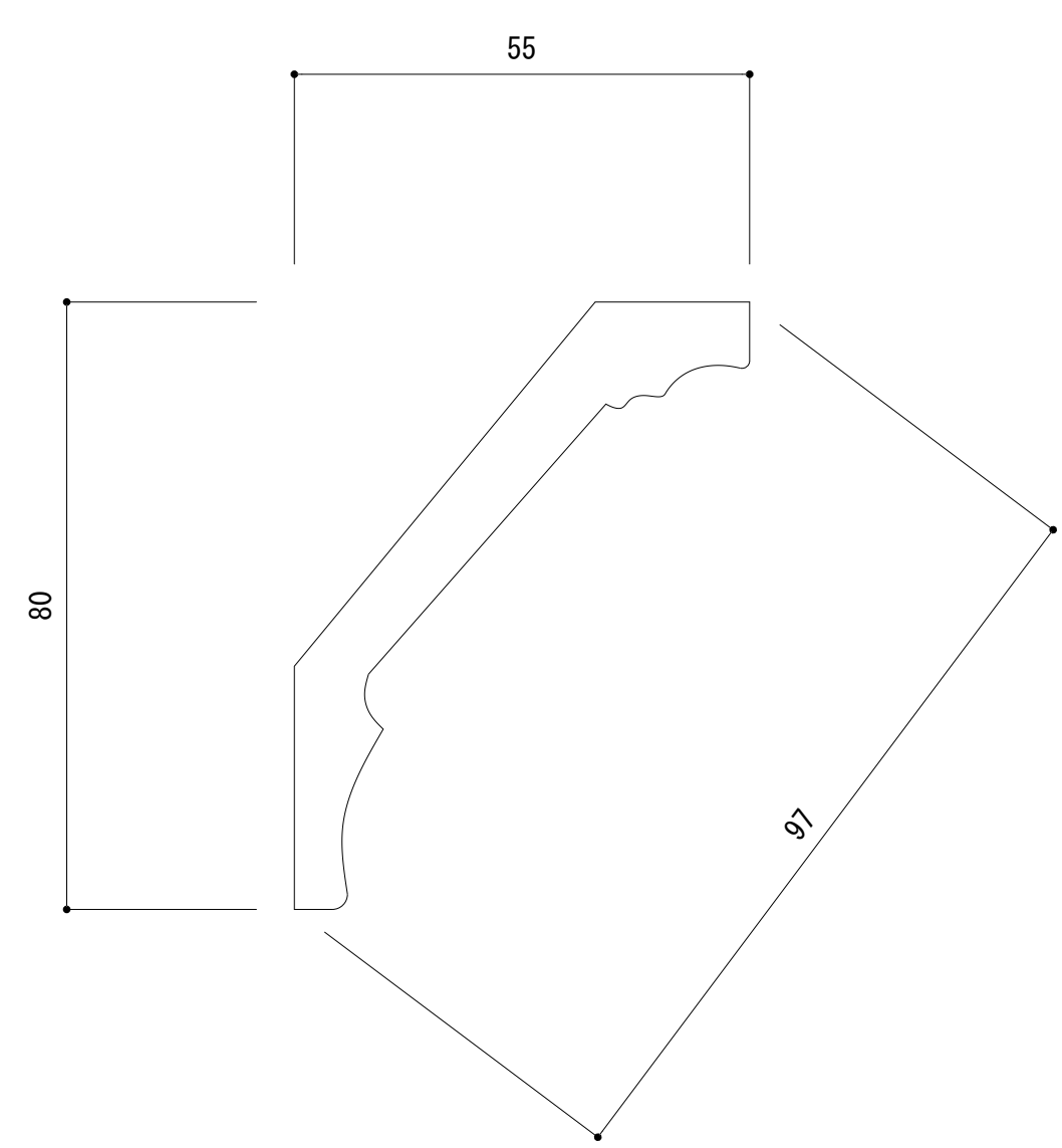
NMG004 80×55×97 ※ ポリウレタン製のため、若干の寸法誤差がある場合があります。
