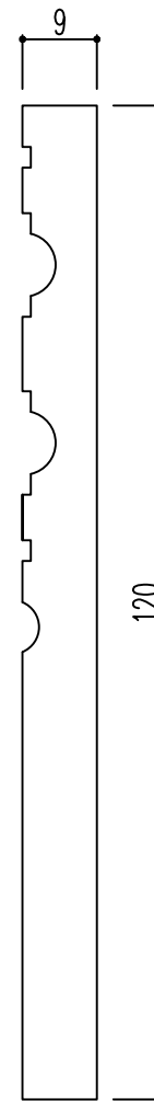
断面図
