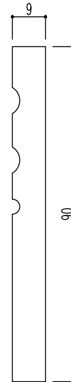
断面図
