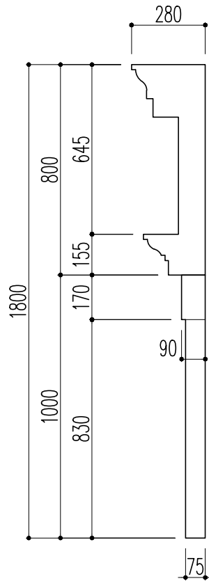
断面図
