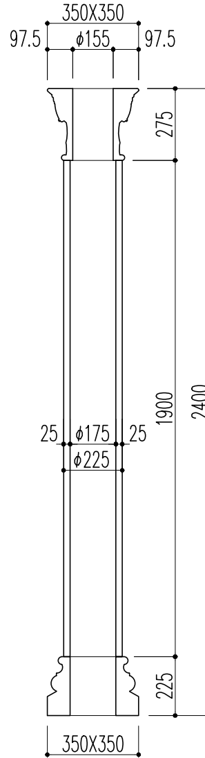
断面図
