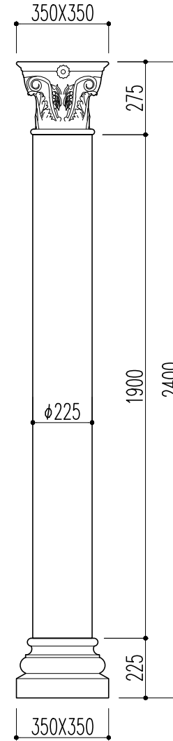
正面図
