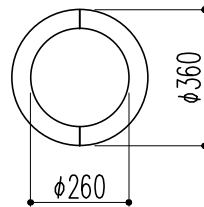
台座断面図 (2分割)
