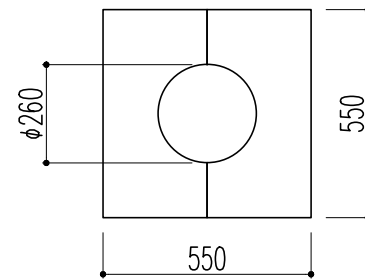
台座断面図 (2分割)
