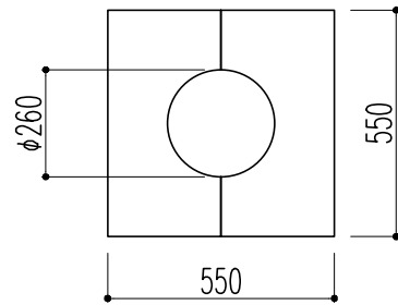
柱頭断面図 (2分割)
