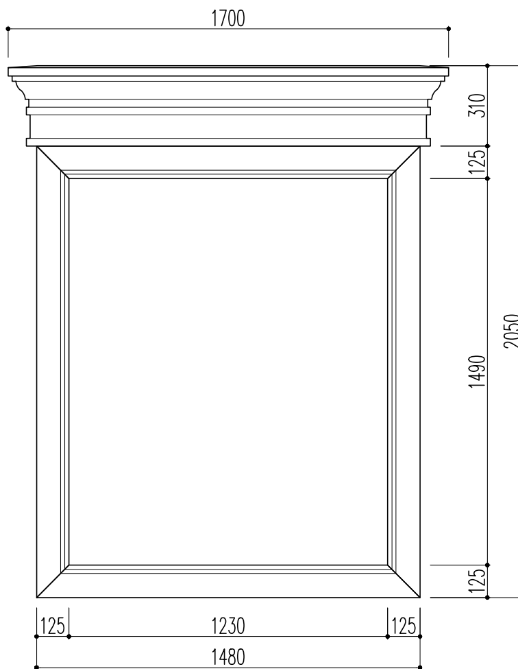
正面図
