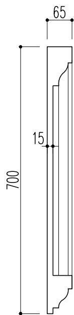
断面図
