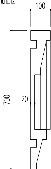
断面図
