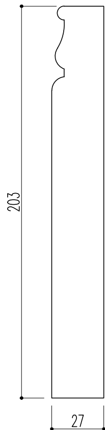
断面図
