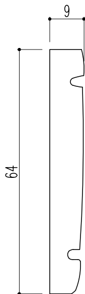
断面図
