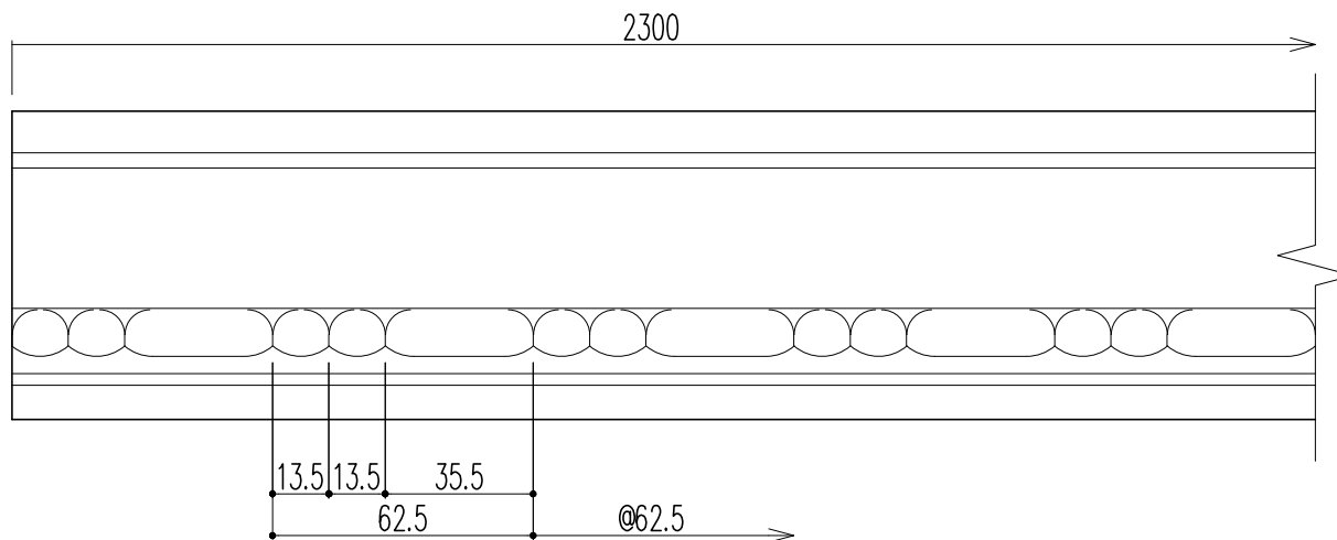
正面図
