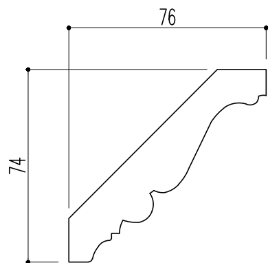
断面図
