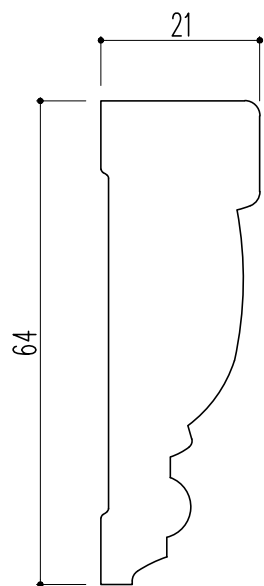
断面図
