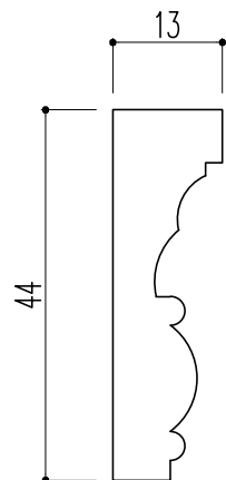
断面図
