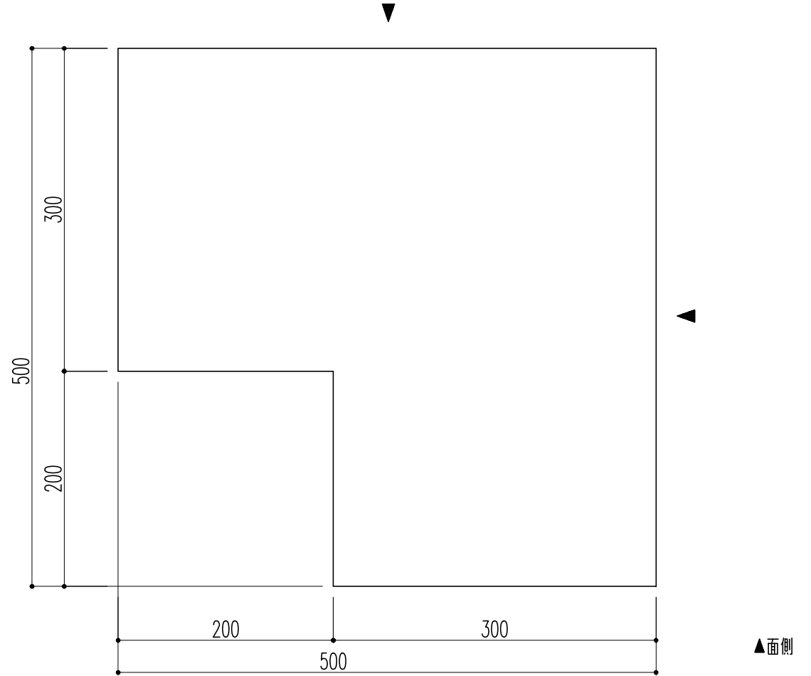
上面図
