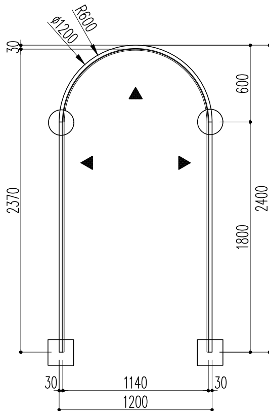
開口枠
