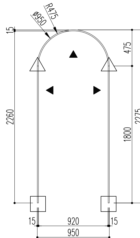
戸当枠
