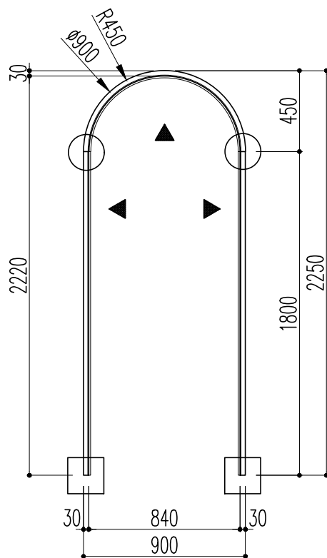
開口枠
