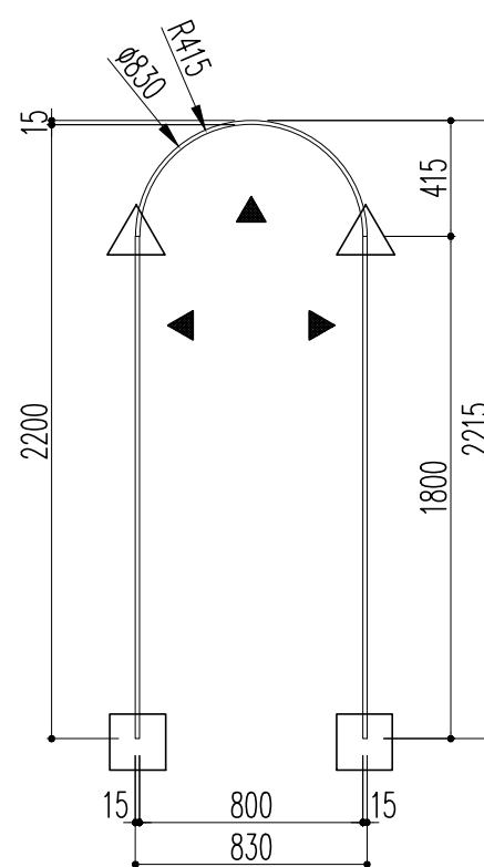
戸当枠
