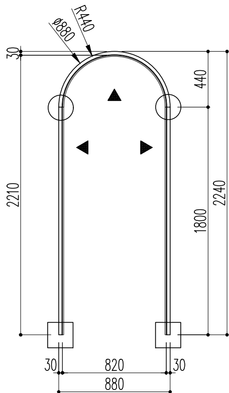
開口枠
