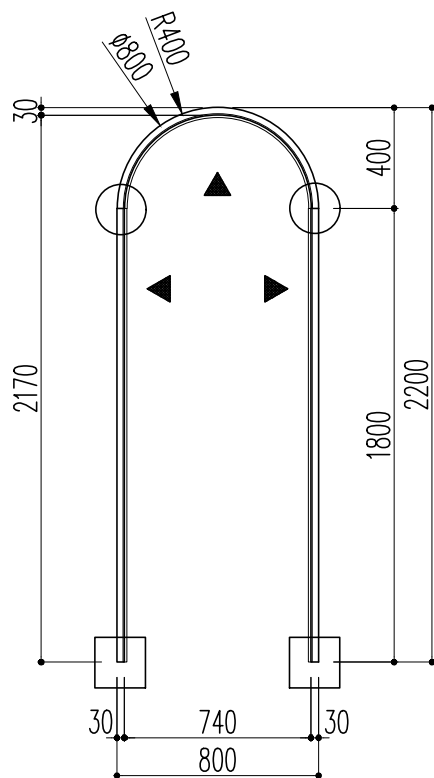
開口枠
