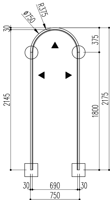
開口枠
