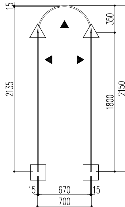
戸当枠
