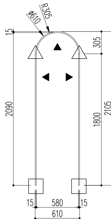
戸当枠
