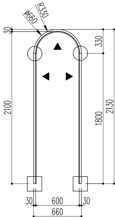
開口枠
