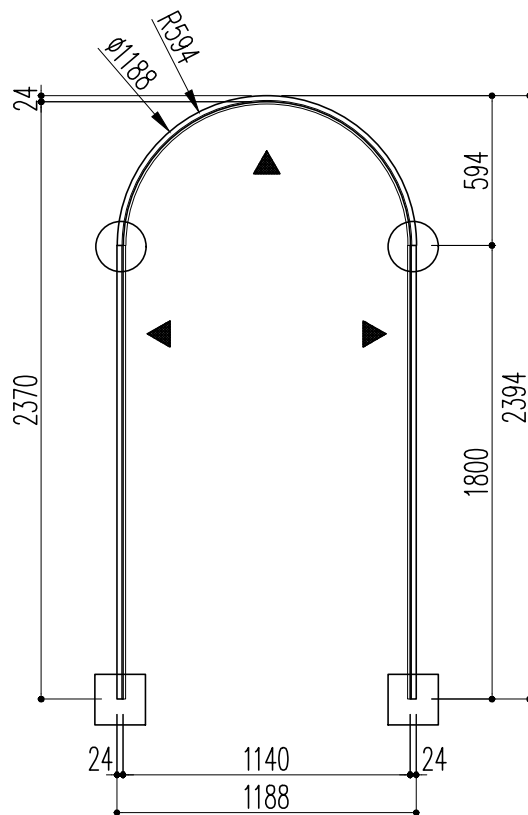
開口枠
