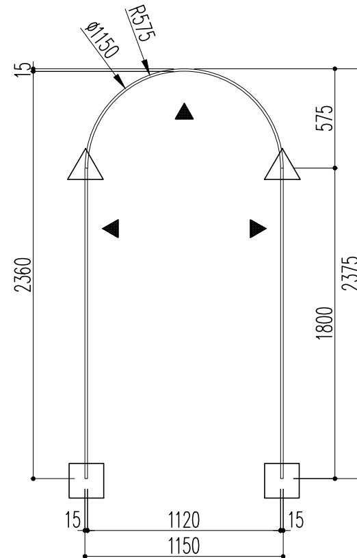
戸当枠
