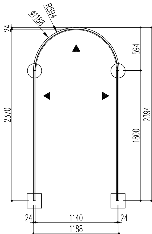
開口枠
