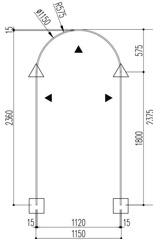
戸当枠
