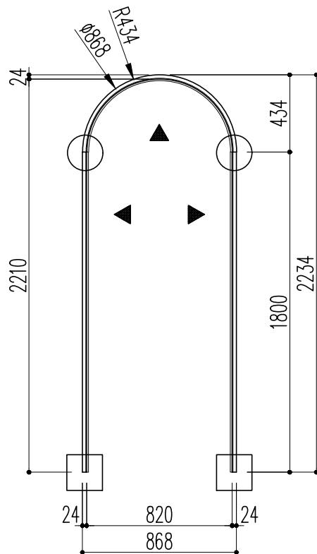
開口枠
