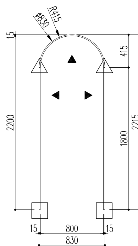
戸当枠
