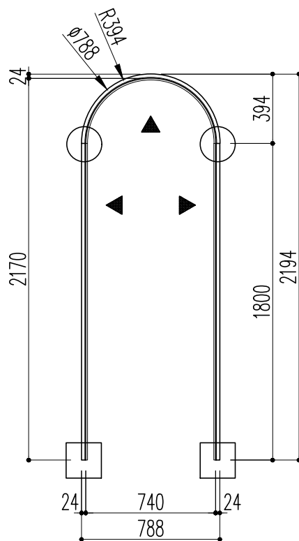
開口枠
