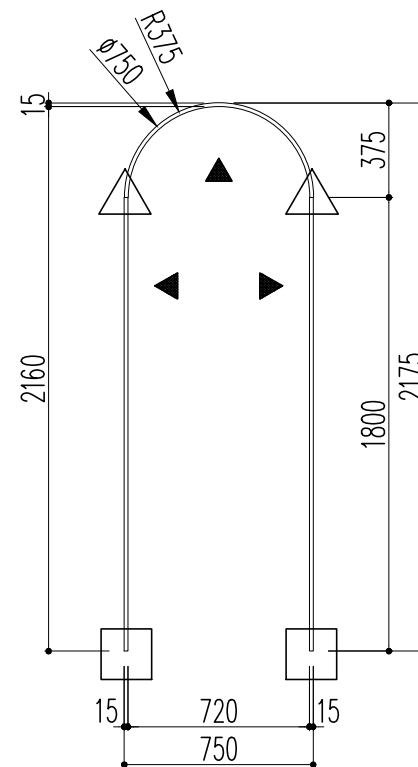
戸当枠
