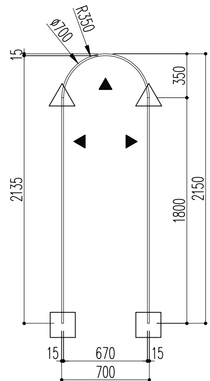
戸当枠
