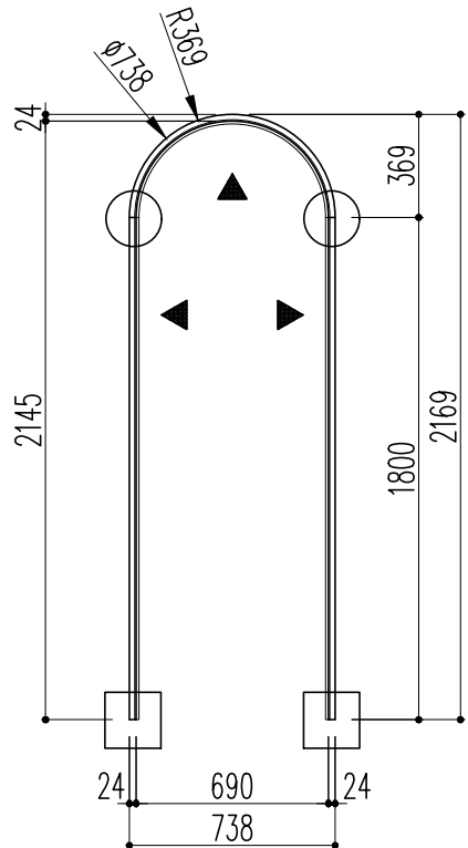
開口枠
