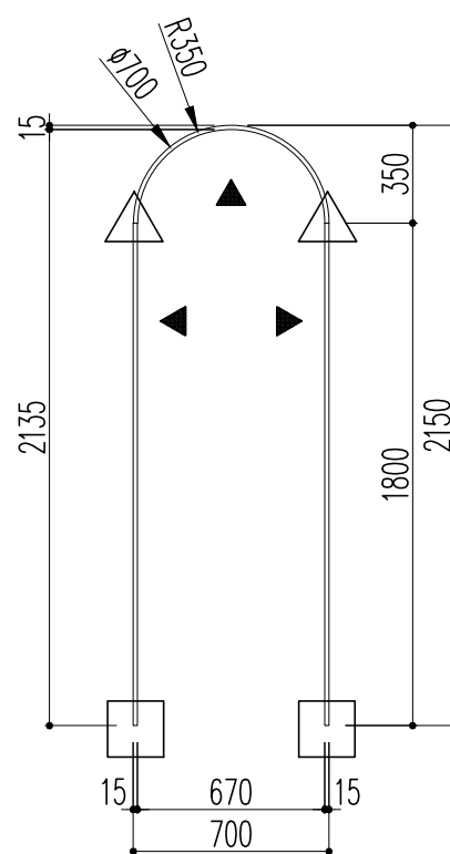
戸当枠
