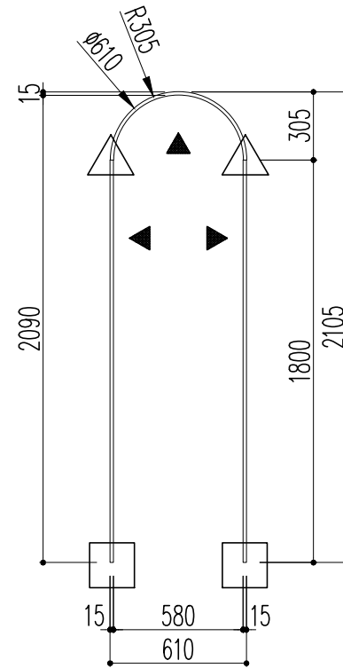
戸当枠
