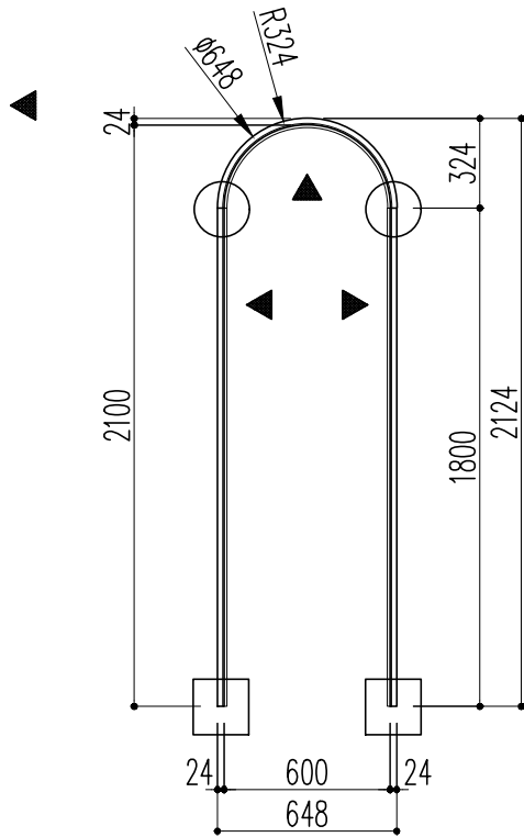
開口枠
