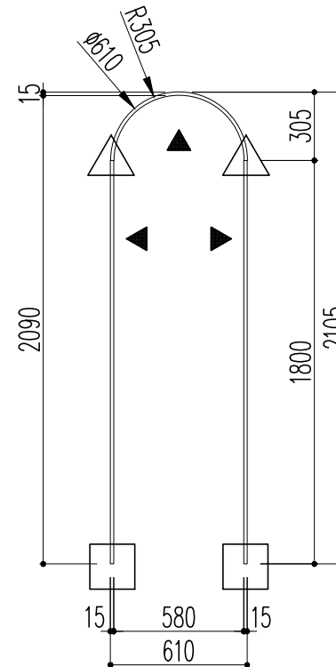
戸当枠
