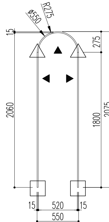
戸当枠
