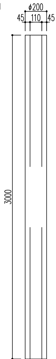
正面図
