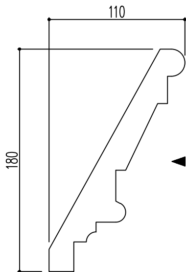
断面図
