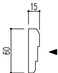
断面図
