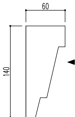
断面図
