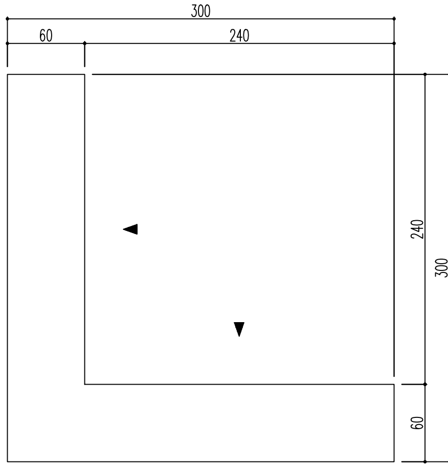
上面図
