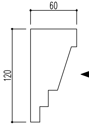
断面図
