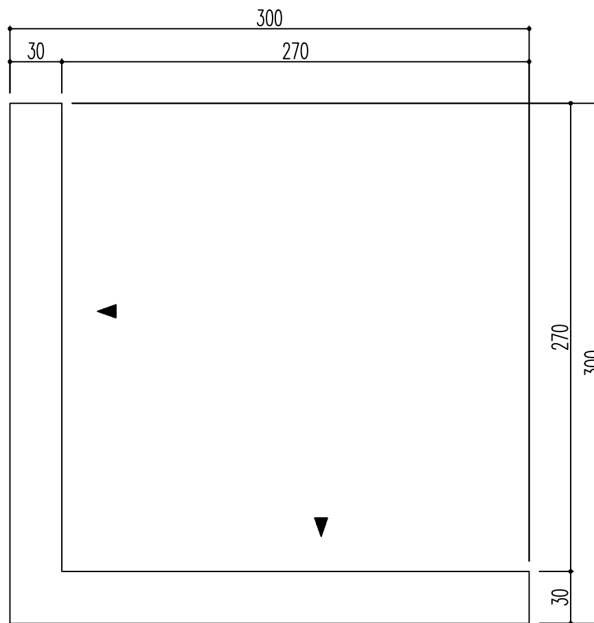
上面図
