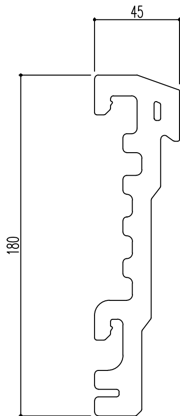
断面図
