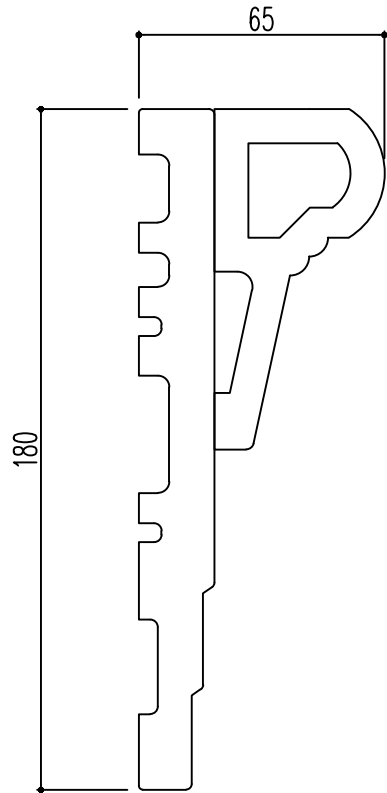
断面図
