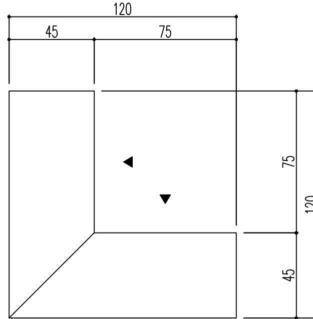
上面図
