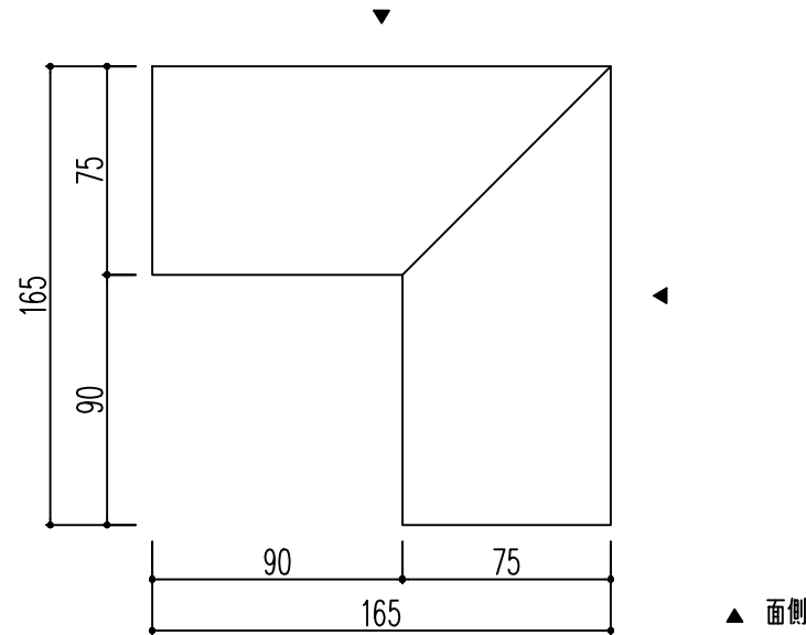
上面図
