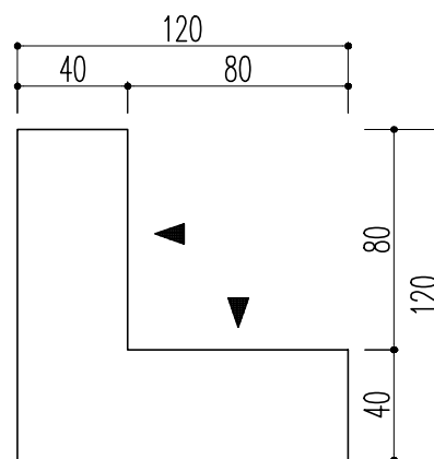
上面図
