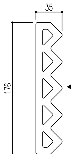
断面図
