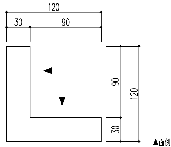
上面図
