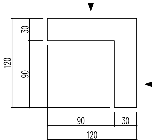
上面図
