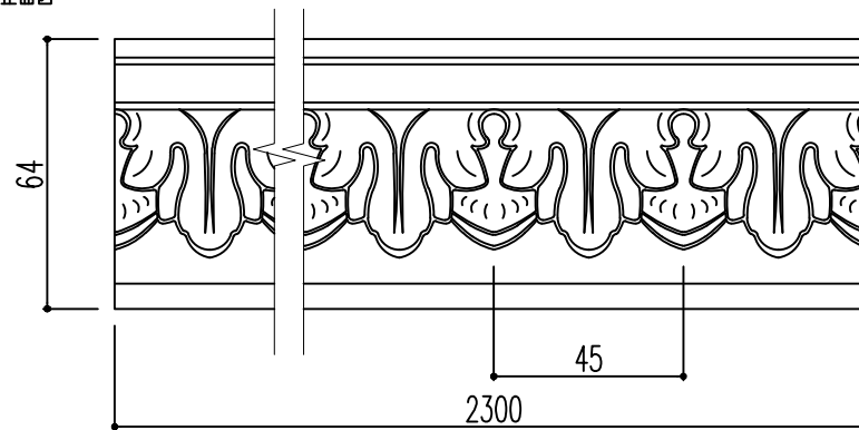
正面図
