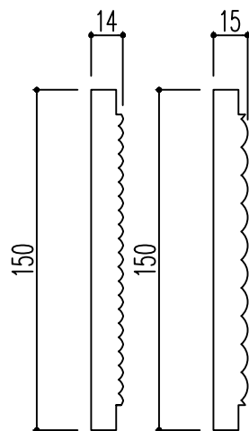
断面図
