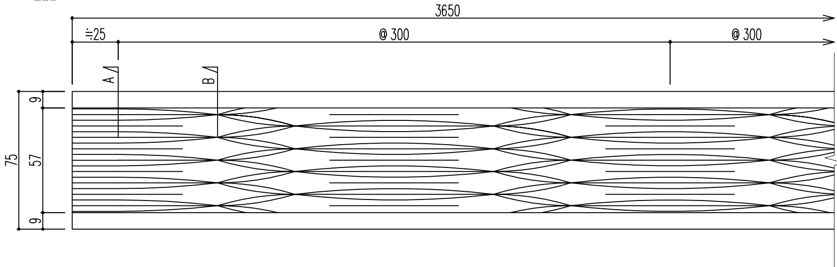
正面図
